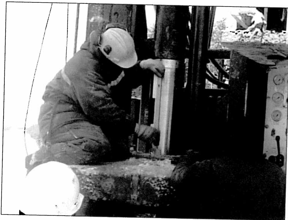
Photographie 4. Aménagement du puits PP-6 en avril 2006.
