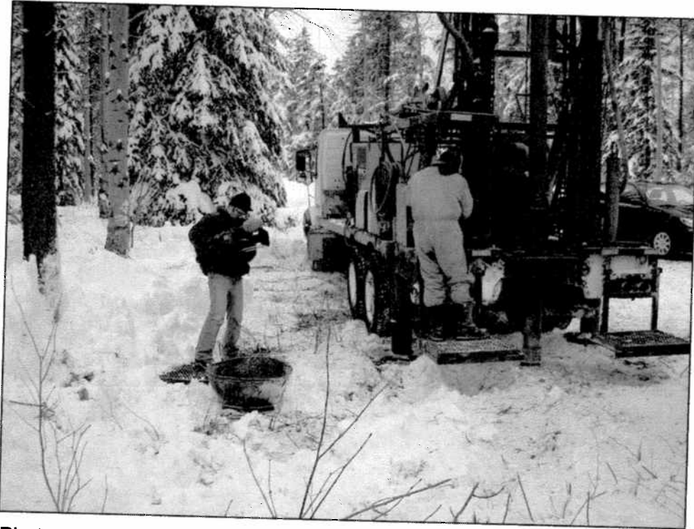
Photographie 1. Forage exploratoire réalisé en février 2006.
